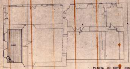
PLANTA DO CORO ESC. 1:100
