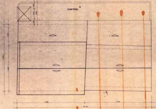
LOCAÇÃO E COBERTURA ESC. 1:100
