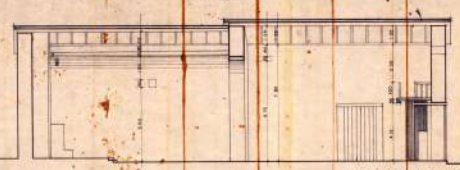
CORTE LONGITUDINAL AA ESC. 1:100
