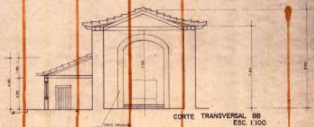
CORTE TRANSVERSAL BB ESC. 1:100
